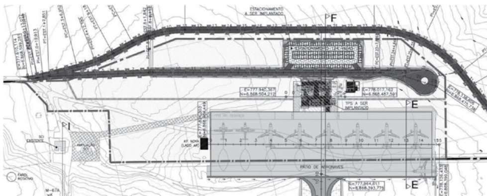
Planta geral AP
