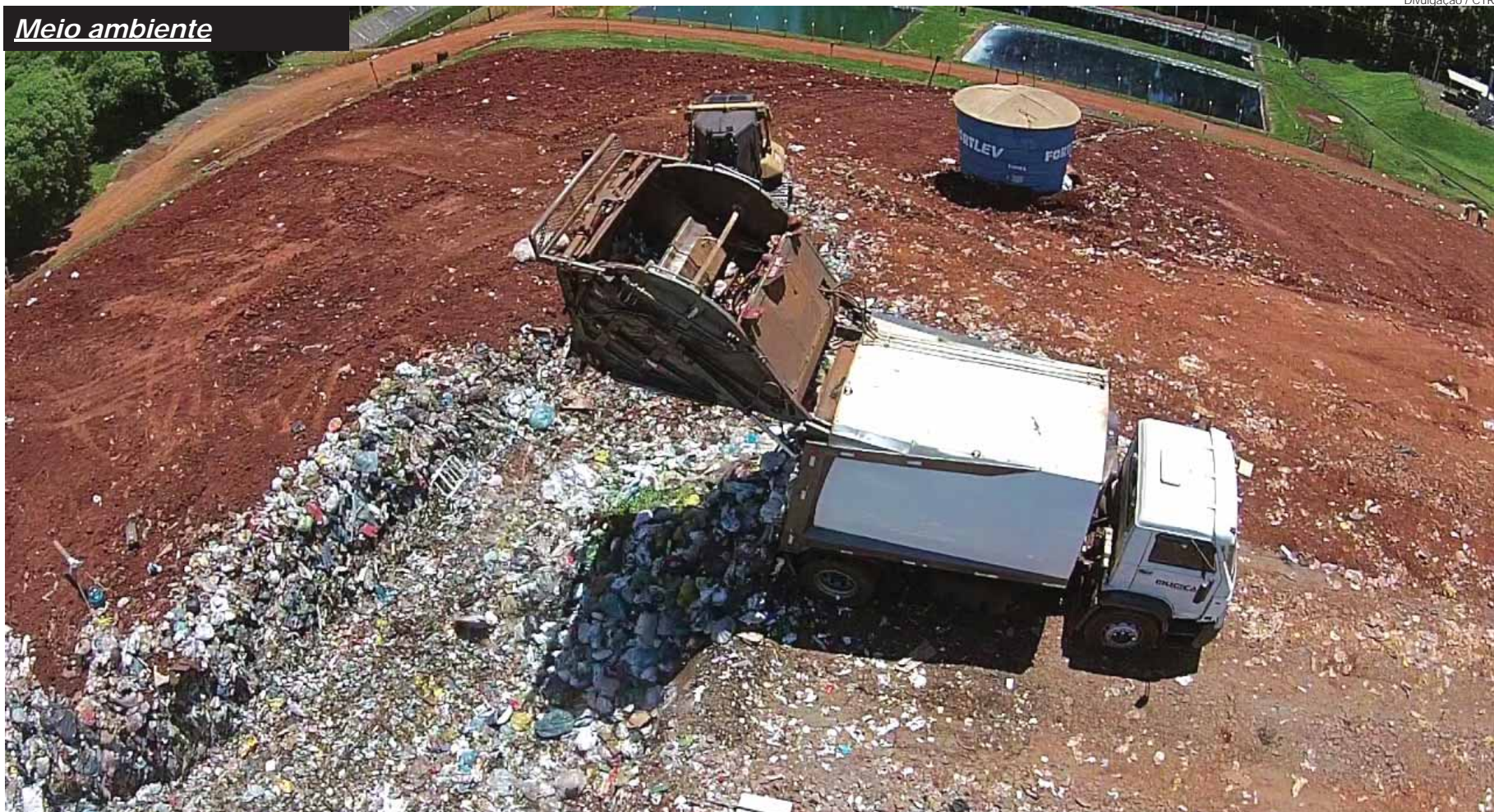
Central de Tratamento de Resíduos (CTR) está instalada em uma área de 20 hectares localizada na cidade de Giruá. A central opera com uma capacidade de 500 toneladas/dia de resíduos, o que permite atender à demanda de toda a região noroeste do estado.
